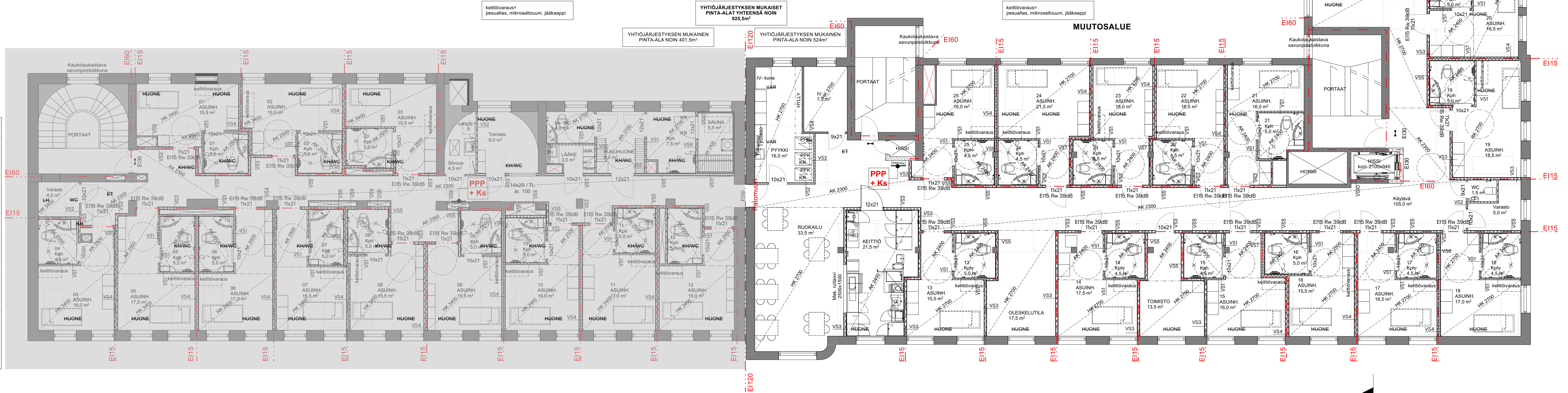
POHJAPIIRUSTUS 4. KERROS 1:100
